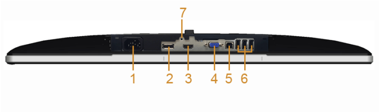
底视图（无显示器支架）
